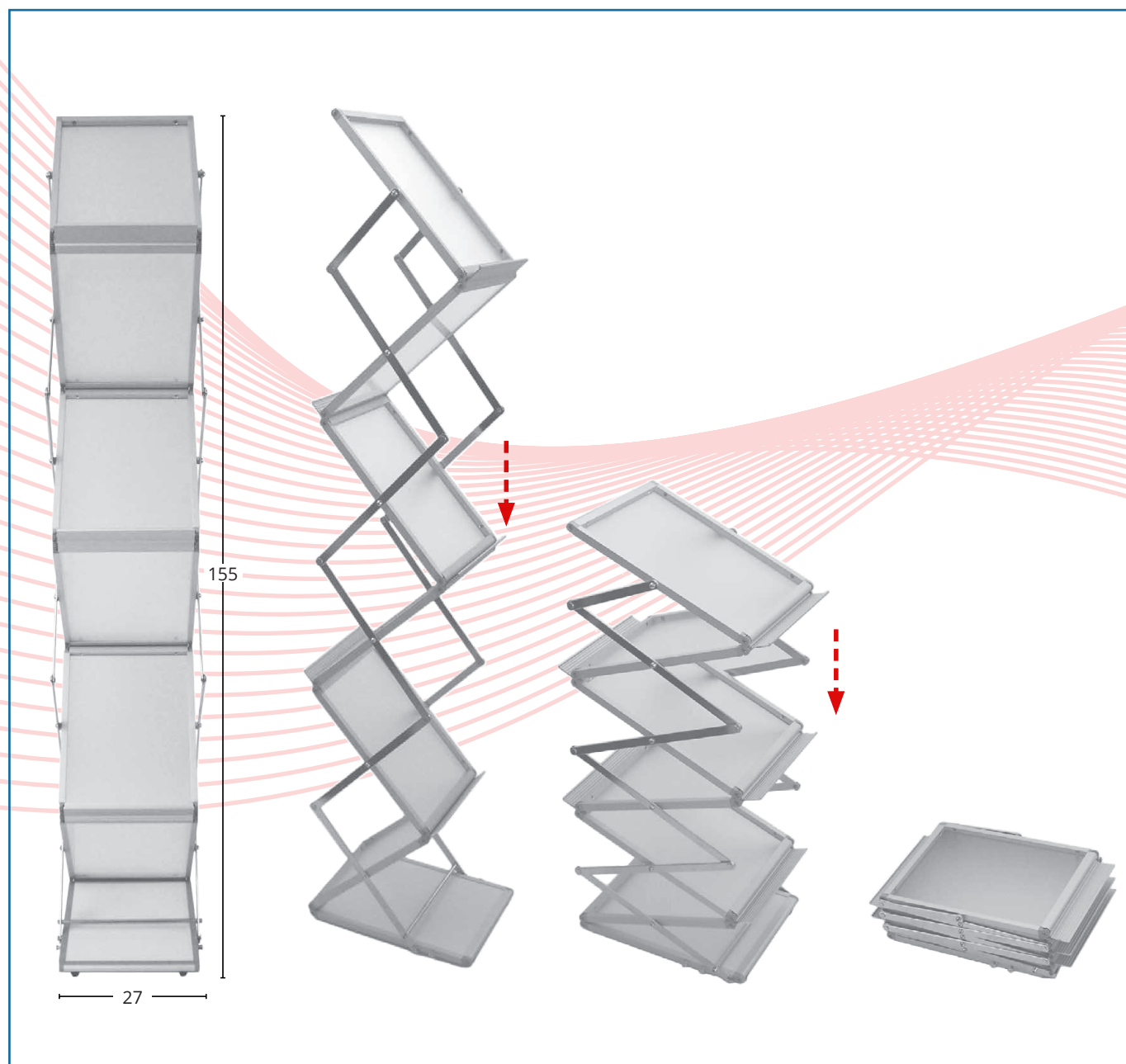
Base personalizzabile in alluminio e opalino, struttura in acciaio e alluminio, 6 piani portadepliant in alluminio e policarbonato.
